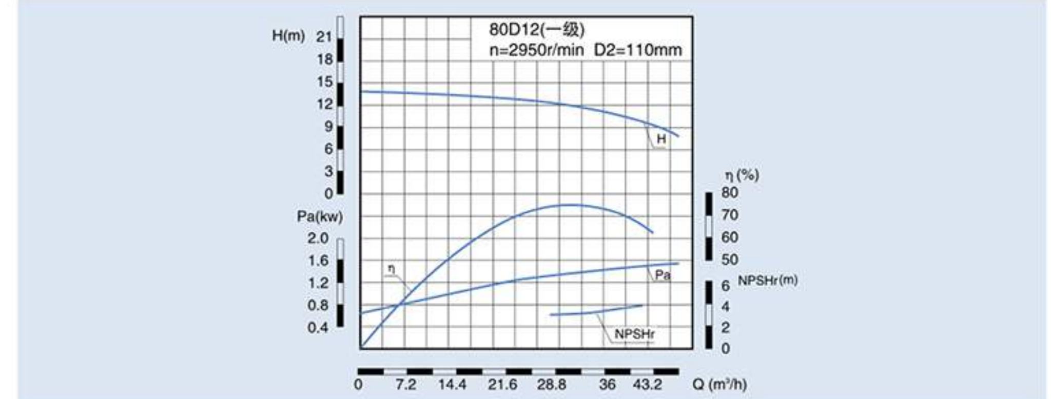
80D、DG、DF、DY、MD12 性能曲线 80D、DG、DF、DY、MD12 Performance Curve
