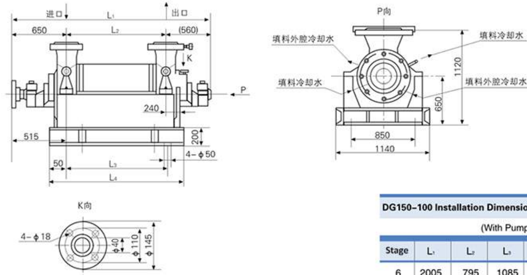
DG150-100型次高压泵外形安装图
