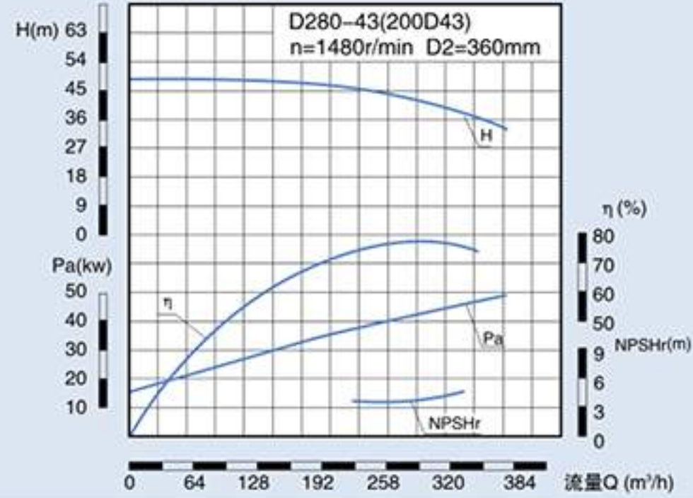
D、DG、DF、DY、MD 280-43(200D43) Performance Data
